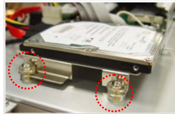
HDD アンチ・バイブレーション機構
